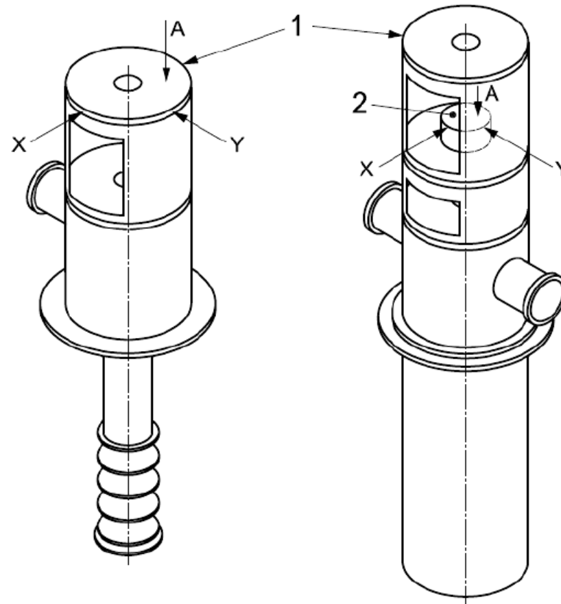
Рисунок 2 - Точки и направления измерений горизонтального насоса
