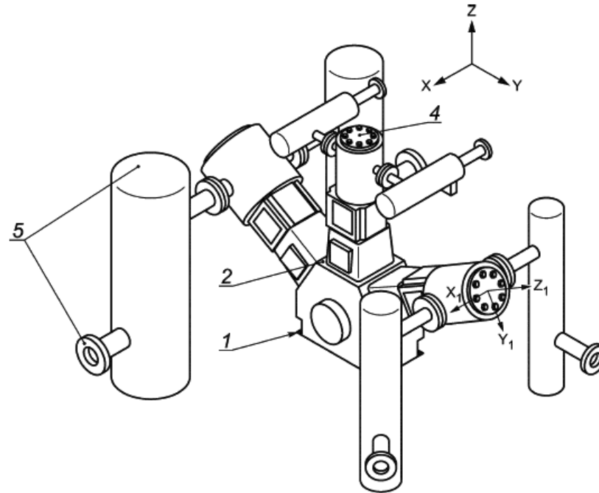
Рисунок 3 - Точки измерений на компрессоре с V-образным расположением цилиндров
