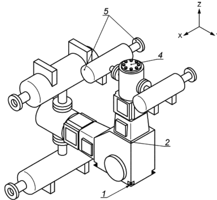
Рисунок 4 - Точки измерений на компрессоре с W-образным расположением цилиндров
