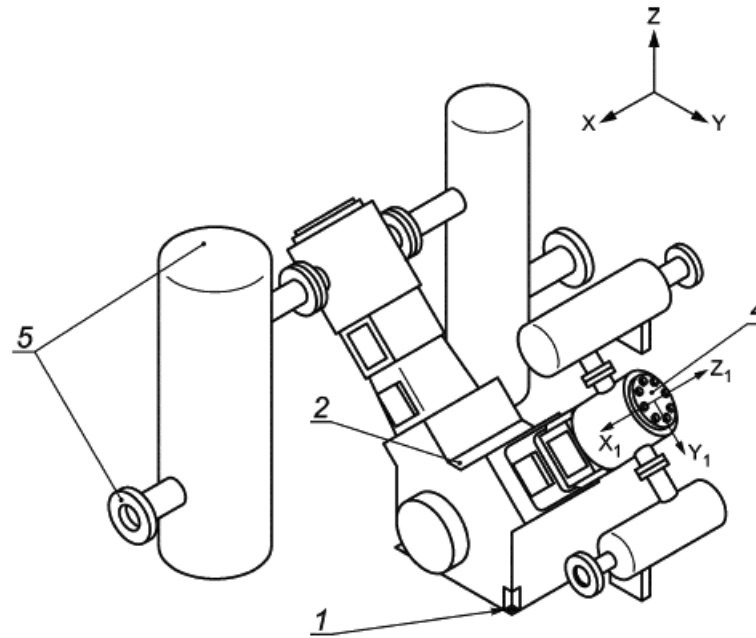
Рисунок 2 - Точки измерений на компрессоре с вертикальным расположением цилиндров
