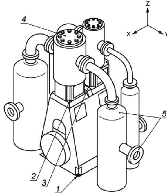
Рисунок 1 - Точки измерений на компрессоре с горизонтальным расположением цилиндров
